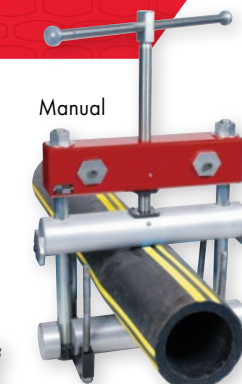
PE Squeeze Tools 8" (225 mm) p. 36 - 38
